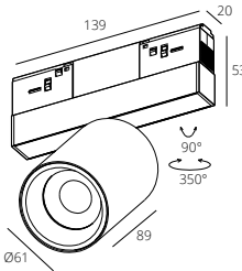
RGD2023/12W
